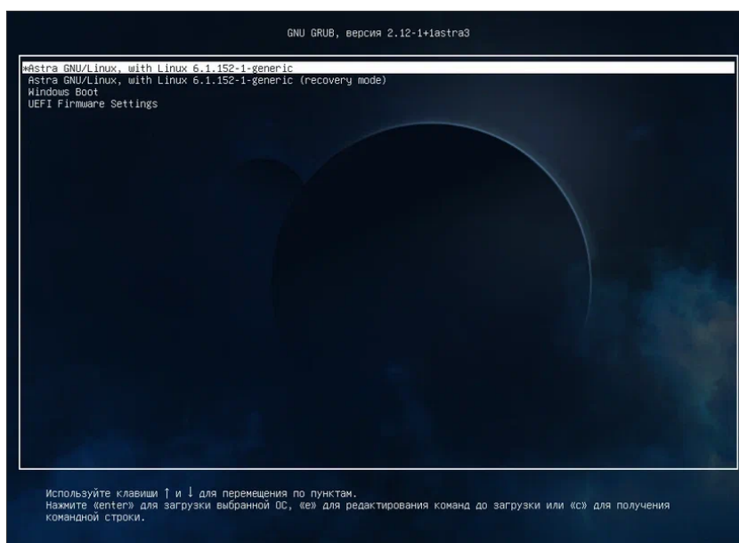
Интерфейс загрузчика
