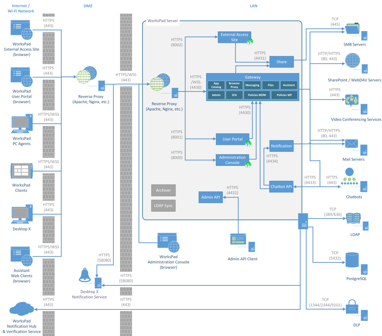
Диаграмма 1. Пример односерверной конфигурации WorksPad.
